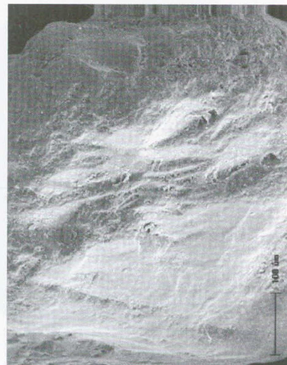
3. Snímky tvaru a povrchu křemenných klastů pomocí SEM. Křemenné klasty frakce 0,5–1 mm; vrstva 1 : a – celkový pohled, b – eolizovaný klast se stopami vodního transportu, c, d – korodovaný povrch se zbytky povlaků v depresích; vrstva 2 : e – celkový pohled, f, g – podélné rýhy způsobené fluvialním transportem.
